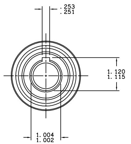
VIEW A-A
