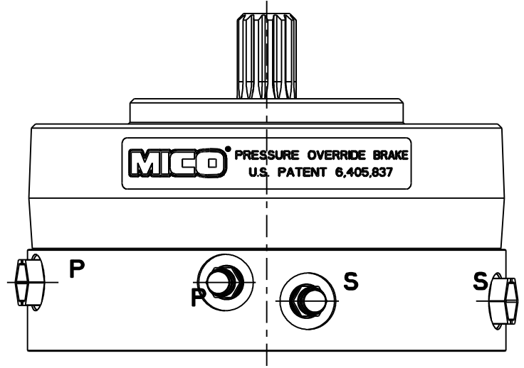
VIEW A-A
